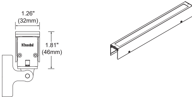
A3- Transversal louver
