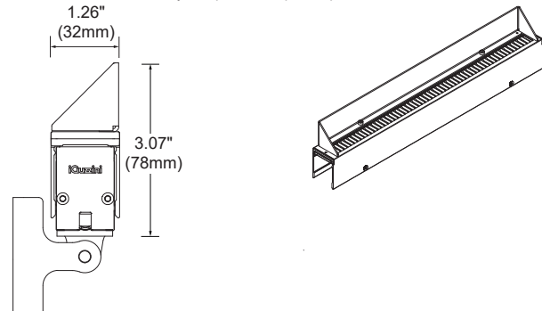
A6- Visor + transversal louver
